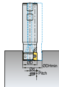
3. Zirkularfräsen einer Durchgangsbohrung
