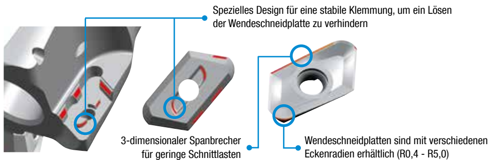
Klemmdesign nach FEM-Analyse Stabile Klemmung der Schneidplatte
