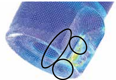
Klemmdesign nach FEM-Analyse Stabile Klemmung der Schneidplatte
